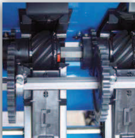
Šestihránný výsevní hřídel s rychlovýměnným zařízením
